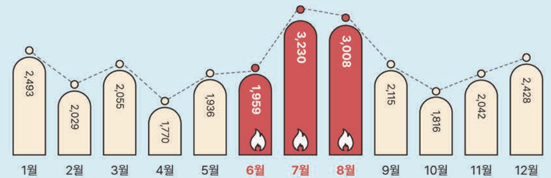
최근 3년간(2023~2025년) 월별 전기화재 현황
